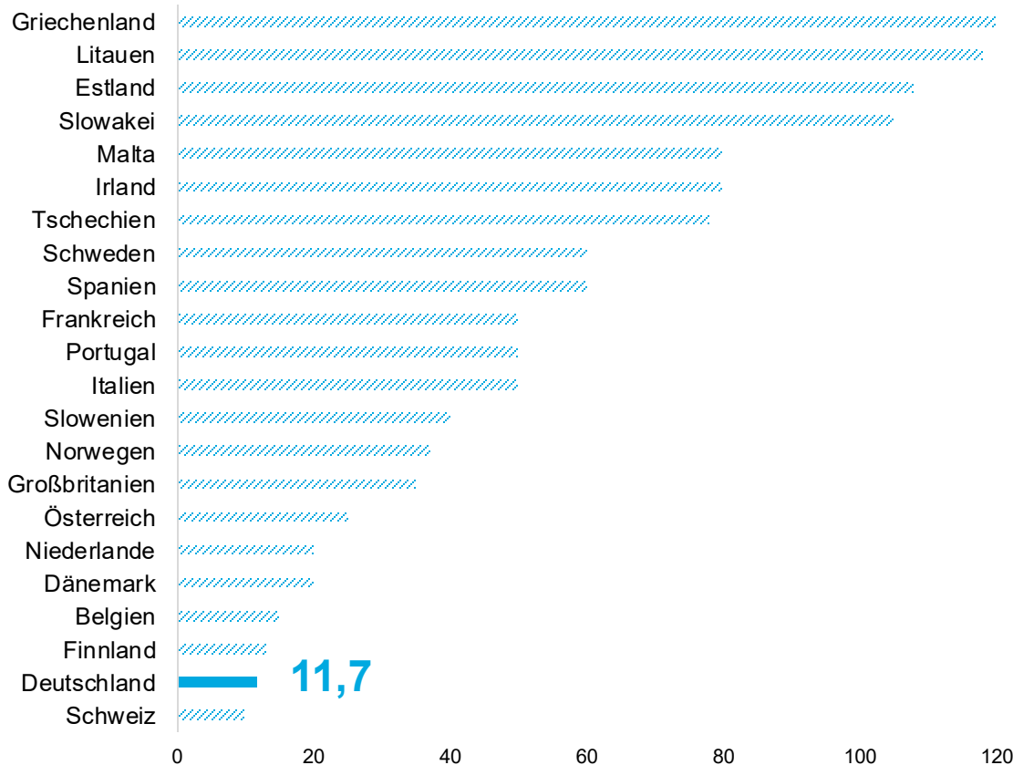
SAIDI Kennzahlen in Minuten pro Jahr
